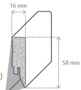
Hartschaum eckig - Grundierfolie weiß RAL 9016 (wasserfest) A0013861/KO42 Maße: 16x58x2400 mm / VPE: 10 Stück
